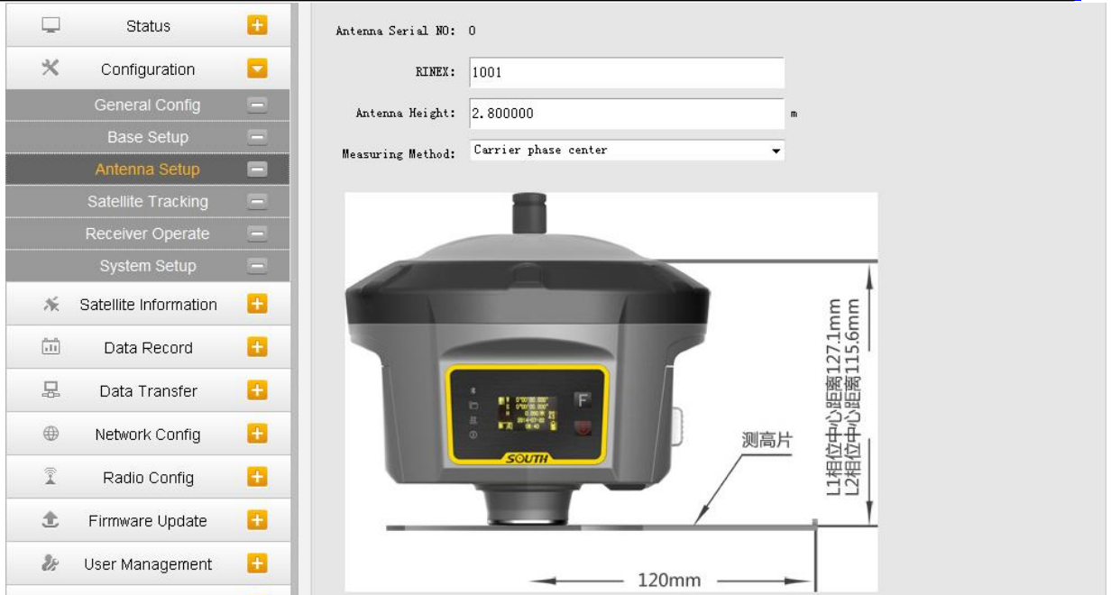
Рисунок 2.3.10 Установка антенны
