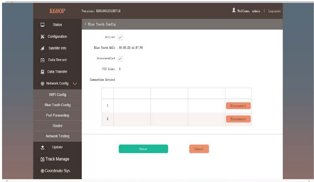
Рисунок 2.3.19 Настройки Bluetooth
