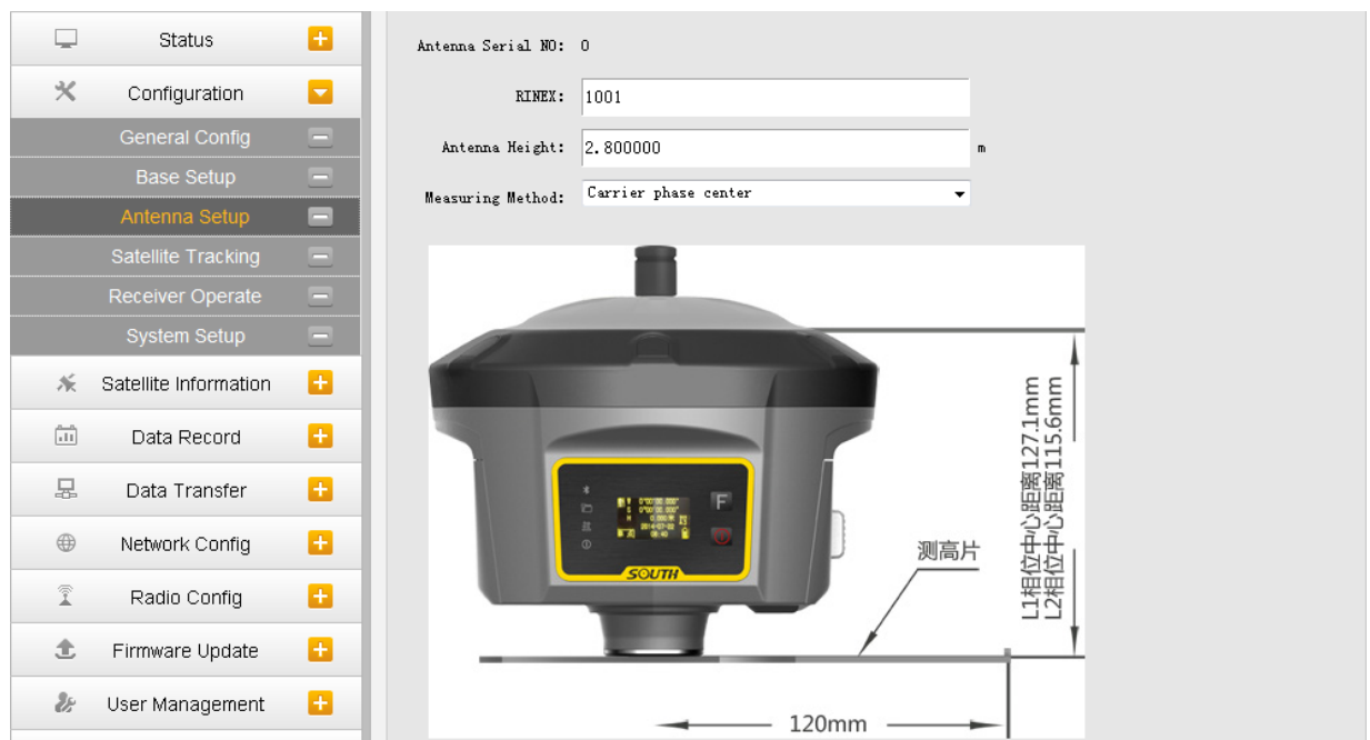
Рисунок 2.3.10 Установка антенны
